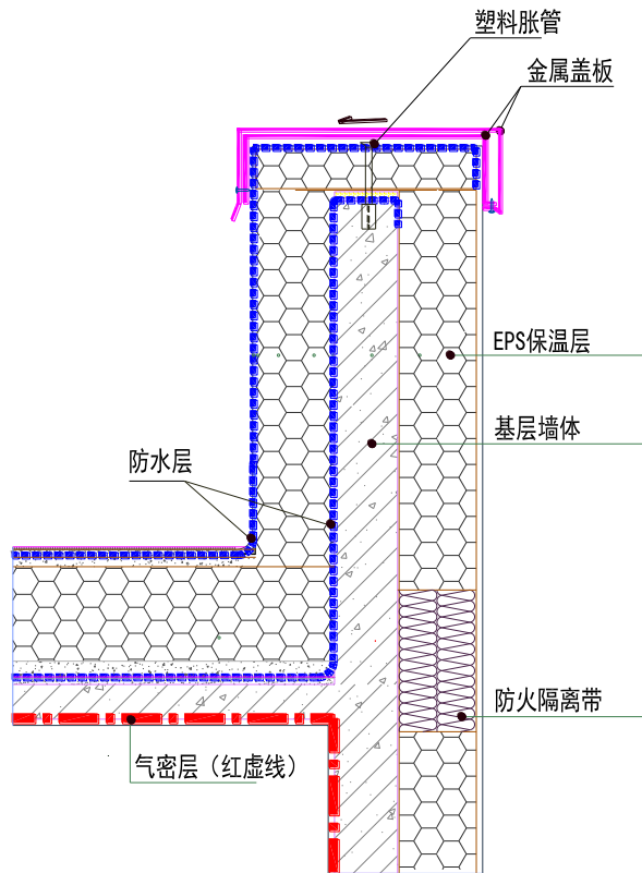
图 3 女儿墙保温做法示意图
