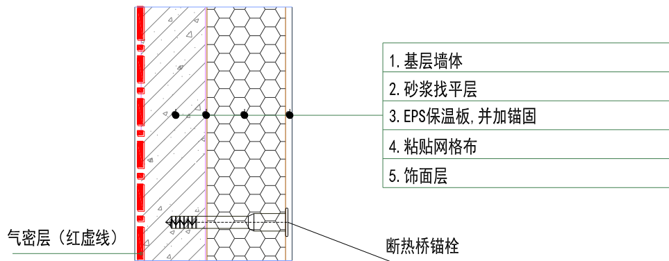
图 1 外墙保温做法示意图
